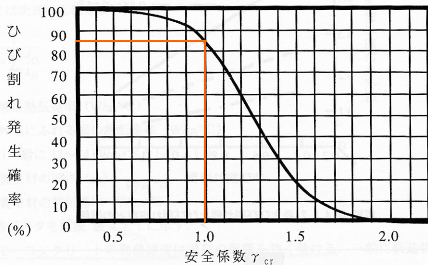
図-4 安全係数とひび割れ発生確率
