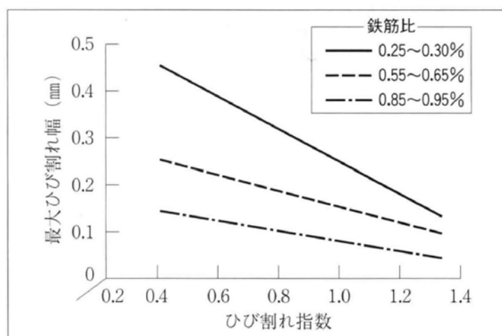
図-6 ひび割れ幅とひび割れ指数との関係
