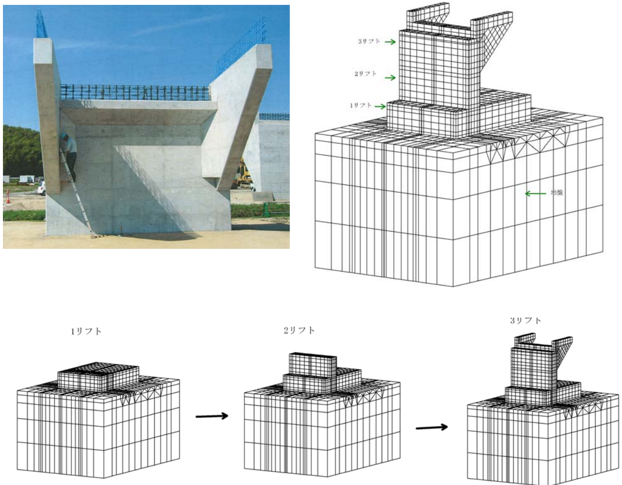
図-1 モデル化
