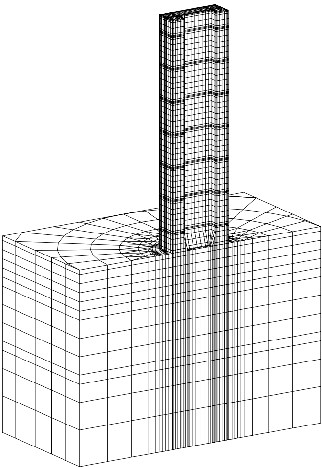
モデル構造図（1/2モデル）
